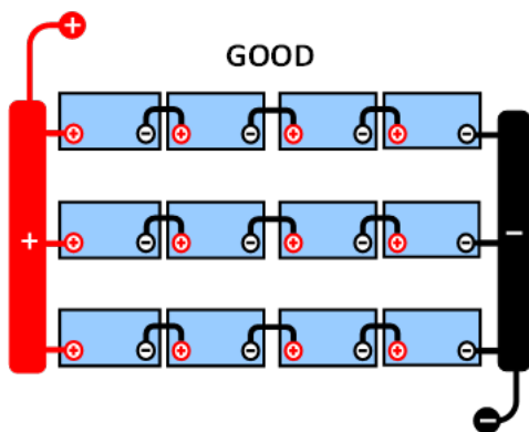
BRA: Mittzonerna är inte anslutna och utan samlingsskenor eller mittzonsövervakning.
