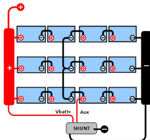
BRA: Mittzonerna är anslutna och med samlingsskenor och mittzonsövervakning.
