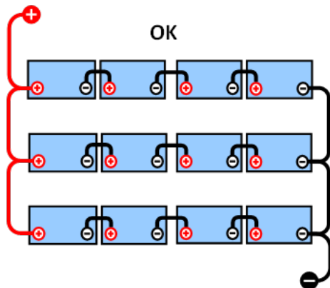
BRA: Mittzonerna är inte anslutna och utan samlingsskenor eller mittzonsövervakning.
