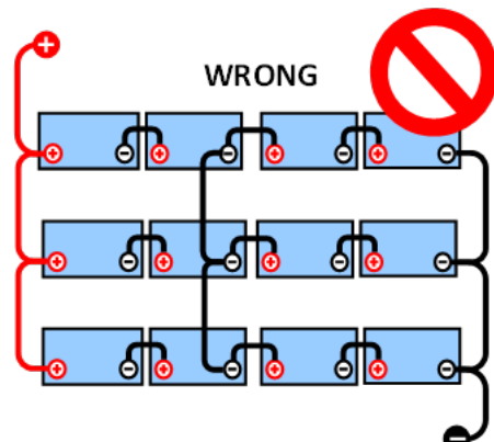
FEL: Mittzonerna är inte anslutna och utan samlingsskenor eller mittzonsövervakning.
